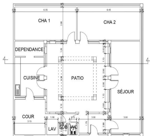
Fig. 07. Vue en plan illustrant l'état initial d'une habitation du village socialiste de Abadla, Source : Auteurs, 2021
