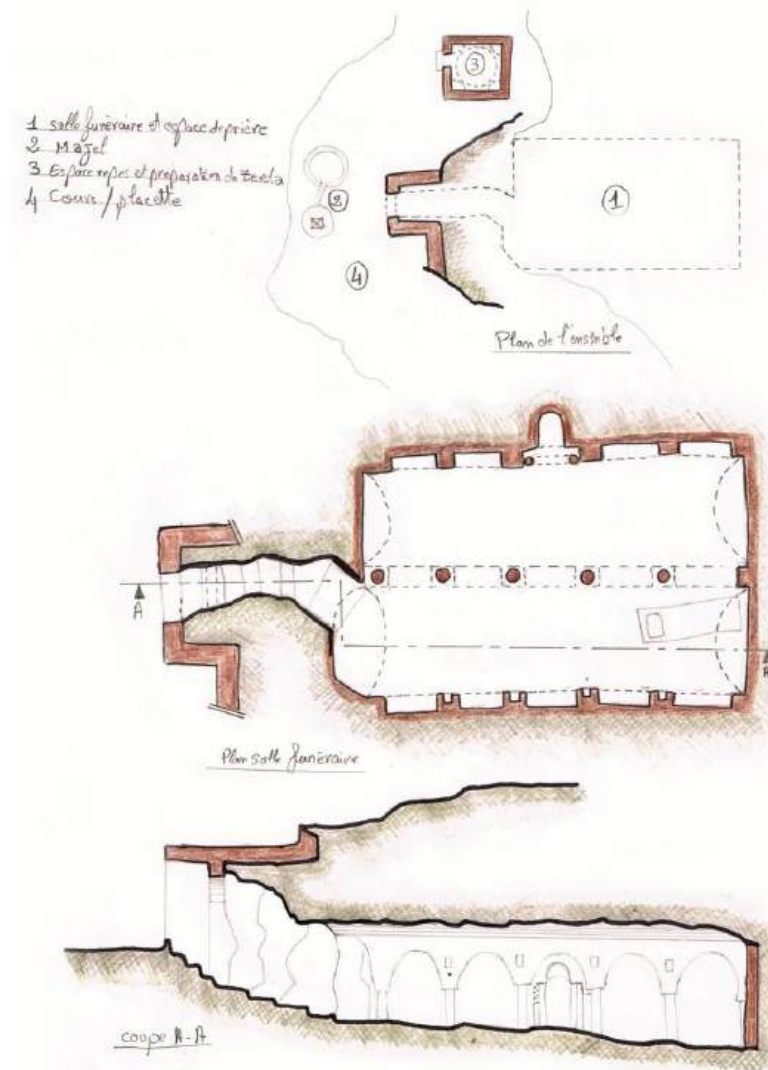
Fig. 48. Plan et coupe de Sidi Ettaj. Réalisation : Asma SEKMANI.
