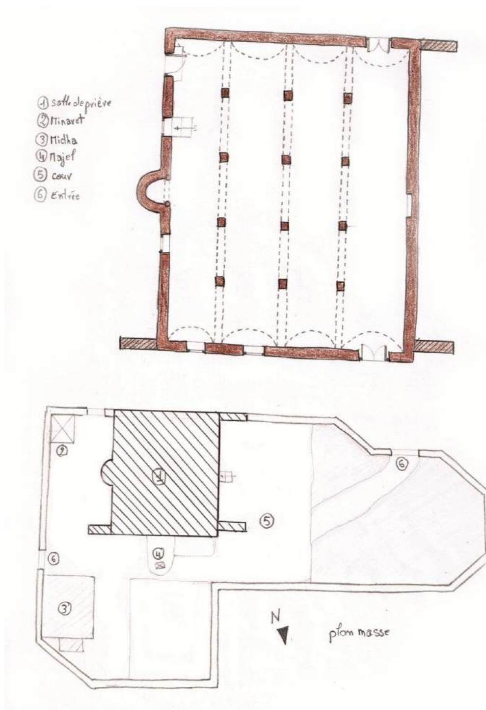
Fig. 43. Plan de la salle de prière et Plan de masse de la mosquée de Essafha. Réalisation : Asma SEKMANI.
