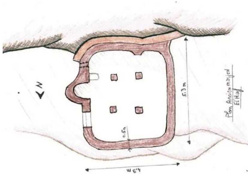
Fig. 36. Plan de l'ancienne mosquée de El-haf. Dessin : Asma SEKMANI.
