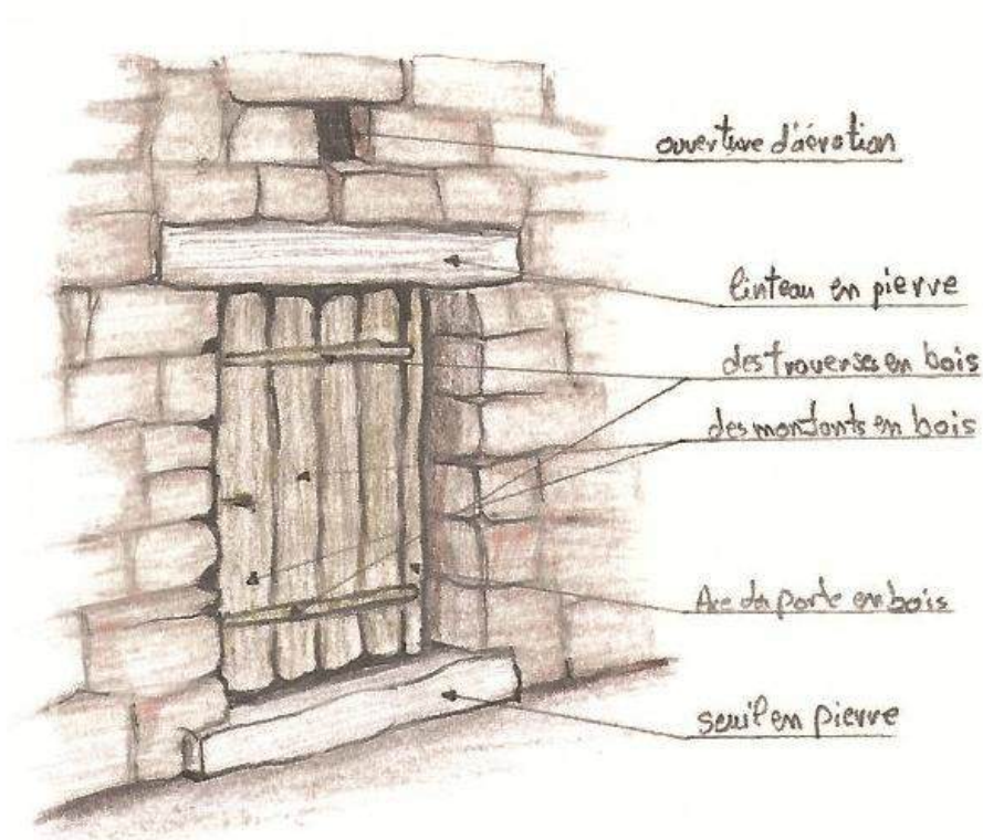
Fig. 87. Façade d'une maison troglodytique à Toujane. Dessin : Asma SEKMANI.
