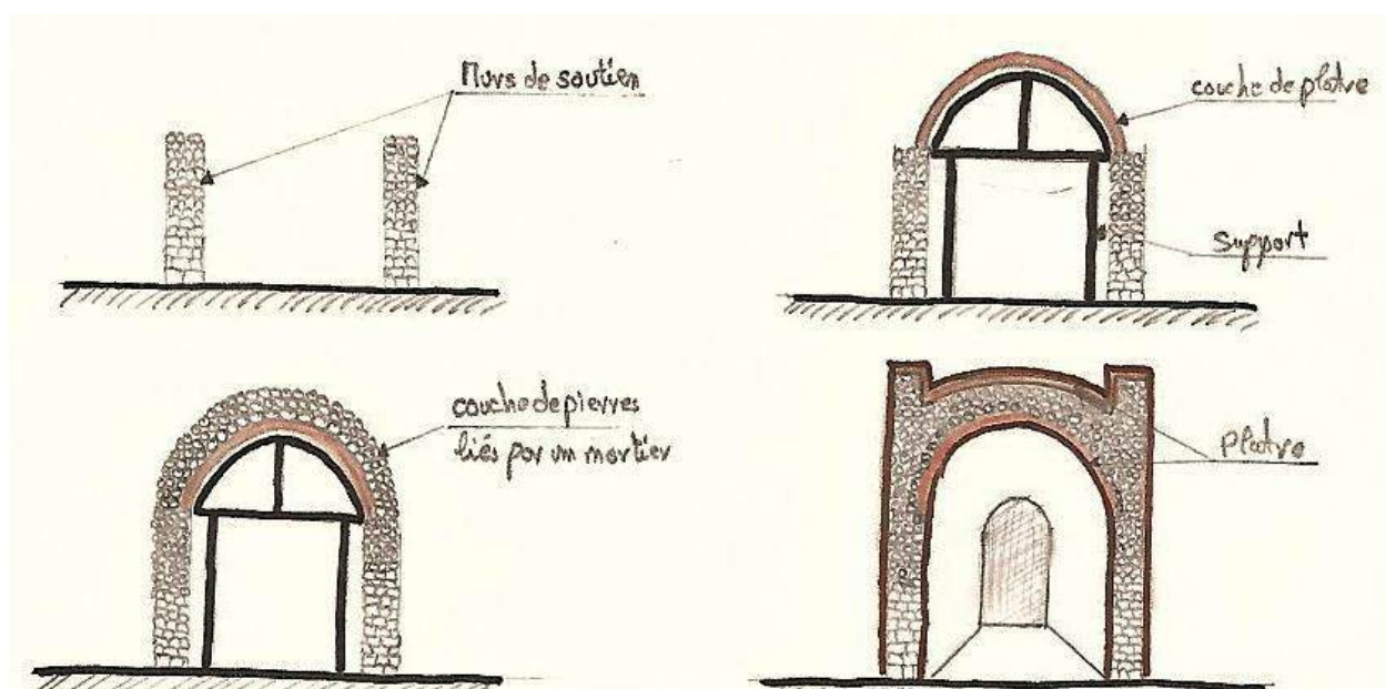
Fig. 85. Dessin : Asma SEKMANI.
