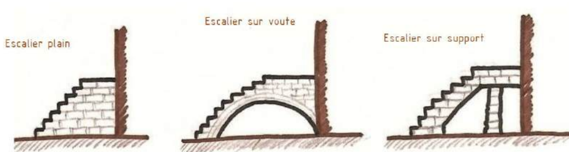
Fig. 89. Exemples des escaliers.
