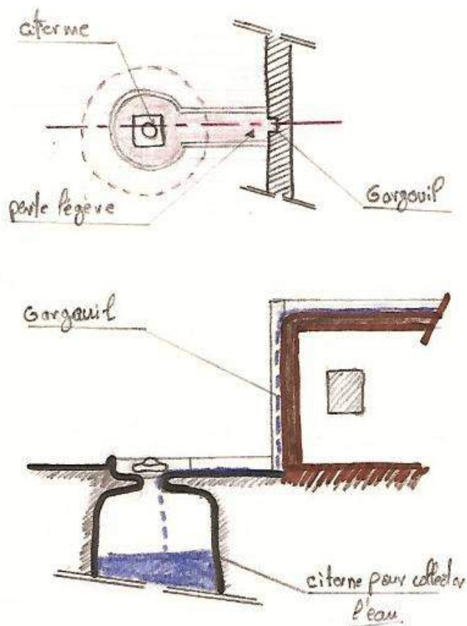
Fig. 90. Majel. Dessin : Asma SEKMANI.
