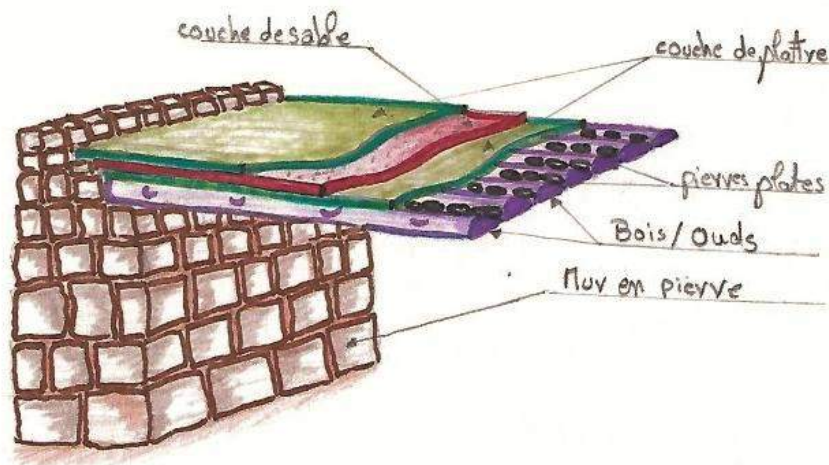
Fig. 83. Toiture.
