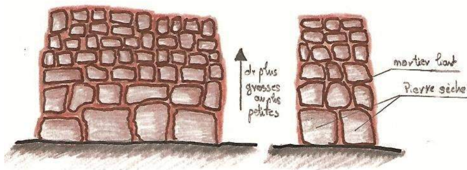
Fig. 79. Croquis Asma SEKMANI.
