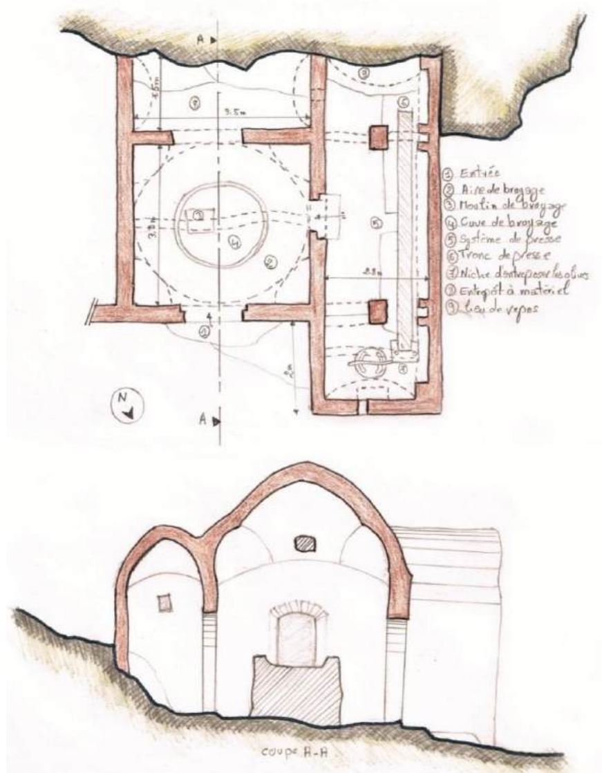
Fig. 52. Plan et coupe d'huilerie Oulad Bourasse. Réalisation : Asma Sekmani.
