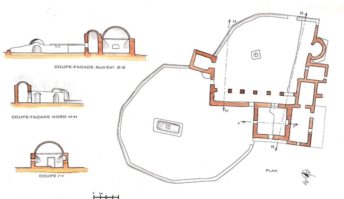
Fig. 8. Relevé du ğama' El koubba en 2004. Source : Dessin de l'auteur.
