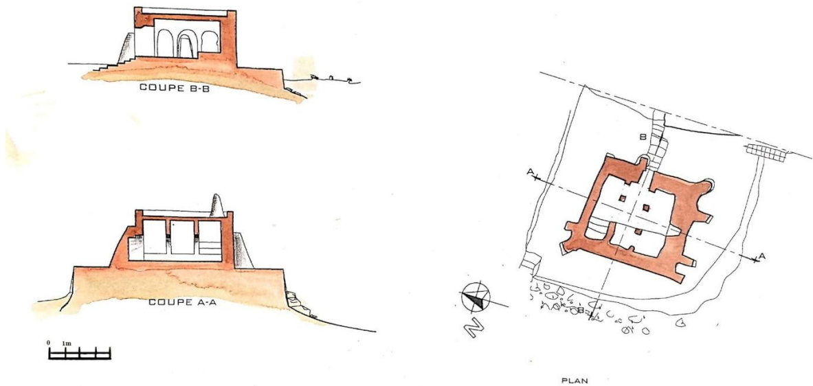
Fig. 2. Relevé du ġama' El fougani en 2004. Source : Dessin de l'auteur.
