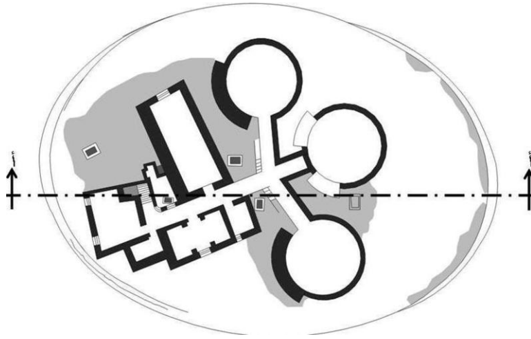
شكل 4 : قطاع أفقي للطابق العلوي لبرج أبو ليلى.
