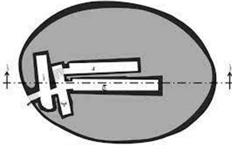
شكل 3 : قطاع أفقي للدور الأرضي لبرج أبو ليلى 57 .
