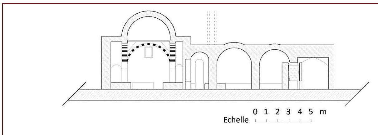
Fig. 15. Coupe A-A Hammam Bou-Sandal. Source : relevé et dessiné par l'auteur.
