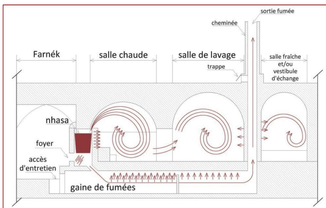
Fig. 13. Transmission de la chaleur de la salle de chaudière vers les salles du Hammam. Source : dessin de l'auteur.
