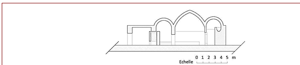
Fig. 19. Coupe B-B du plan de Hammam el-Marr. Source : relevé et dessiné par l'auteur.
