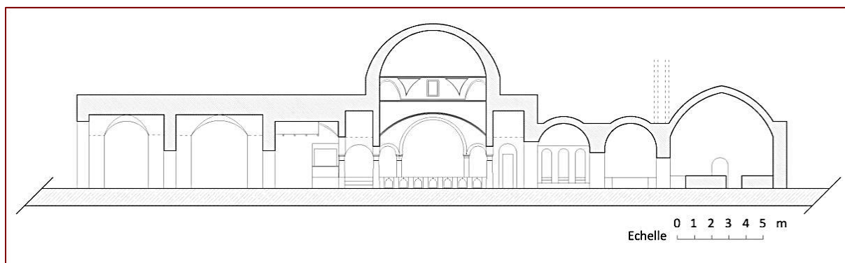
Fig. 18. Coupe A-A du plan de Hammam el-Marr. Source : relevé et dessiné par l'auteur.
