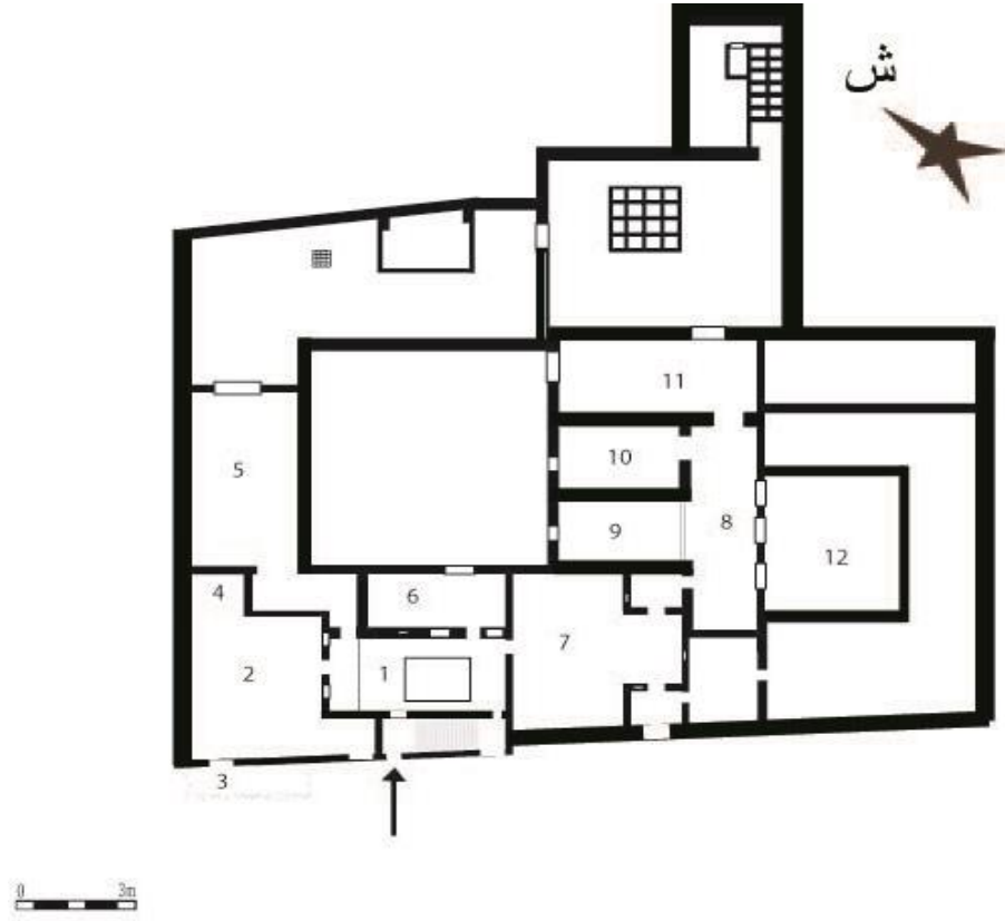
صورة 4. مخطط دار زروق الطابق الثاني (إنجاز منى كمون).
